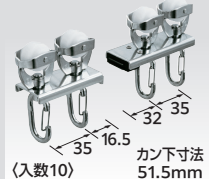
D40マグネットランナー(両開) ワンタッチランナーSタイプ
