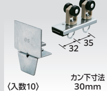
D40片マグネットランナー(片開) ランナーAタイプ
