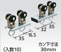
D40マグネットランナー(両開) ランナーAタイプ
