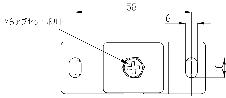
D40扉吊用ランナー (15Y68)
