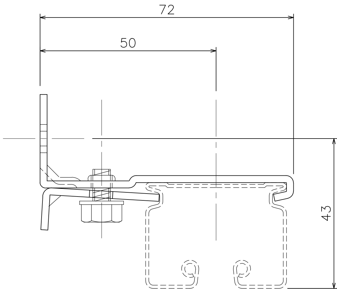
D40 Sブラケット (15T41)
