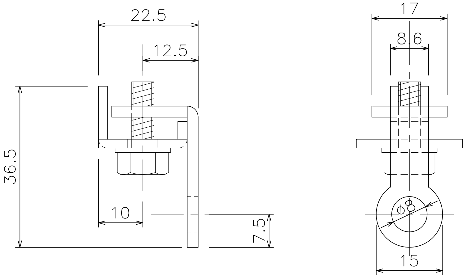
D30 ステン中間ストップ (13T39)
