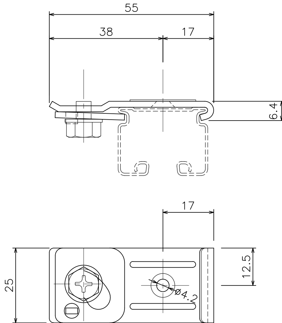
D30 ステン天井Sブラケット (13T51)
