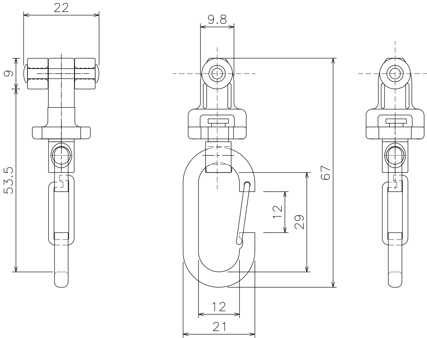
D30 後付ワンタッチランナー (12T20)
