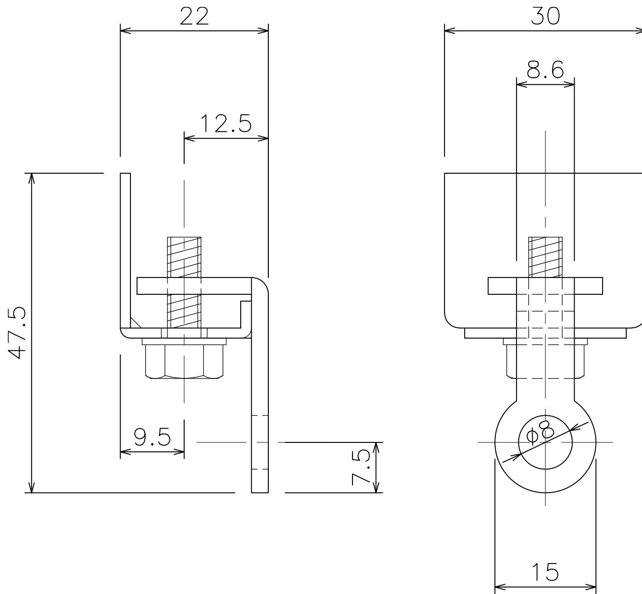
D30 キャップストップ (12T31)
