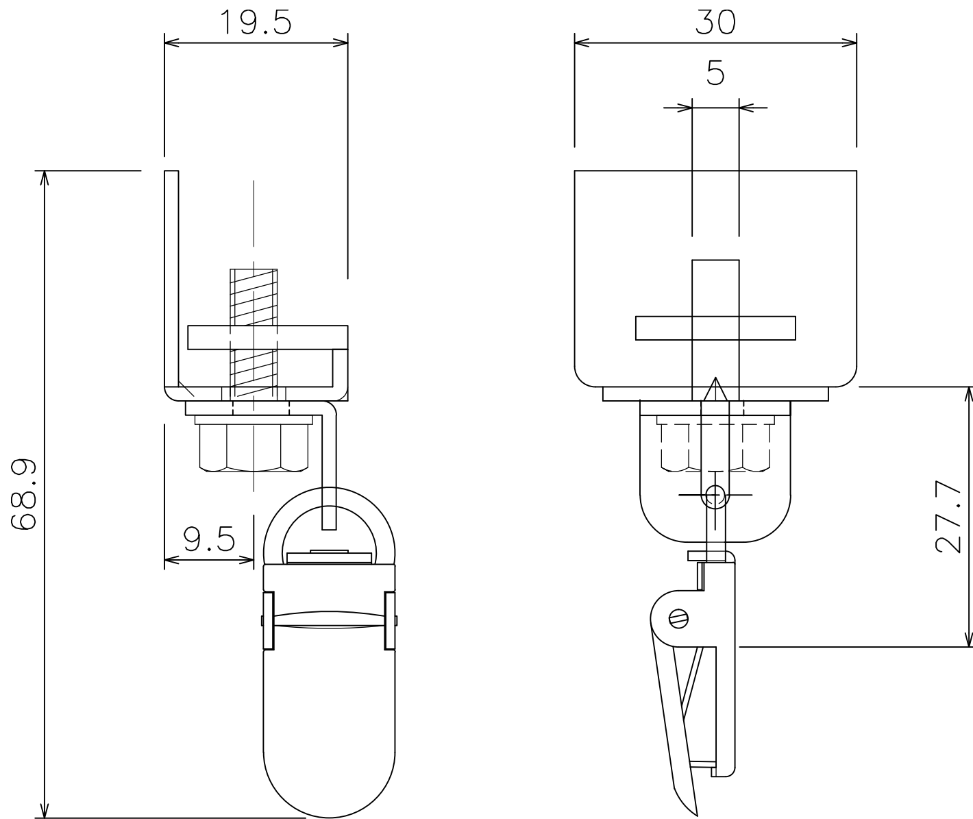
D30 クリッパー付キャップストップ (12T32)
