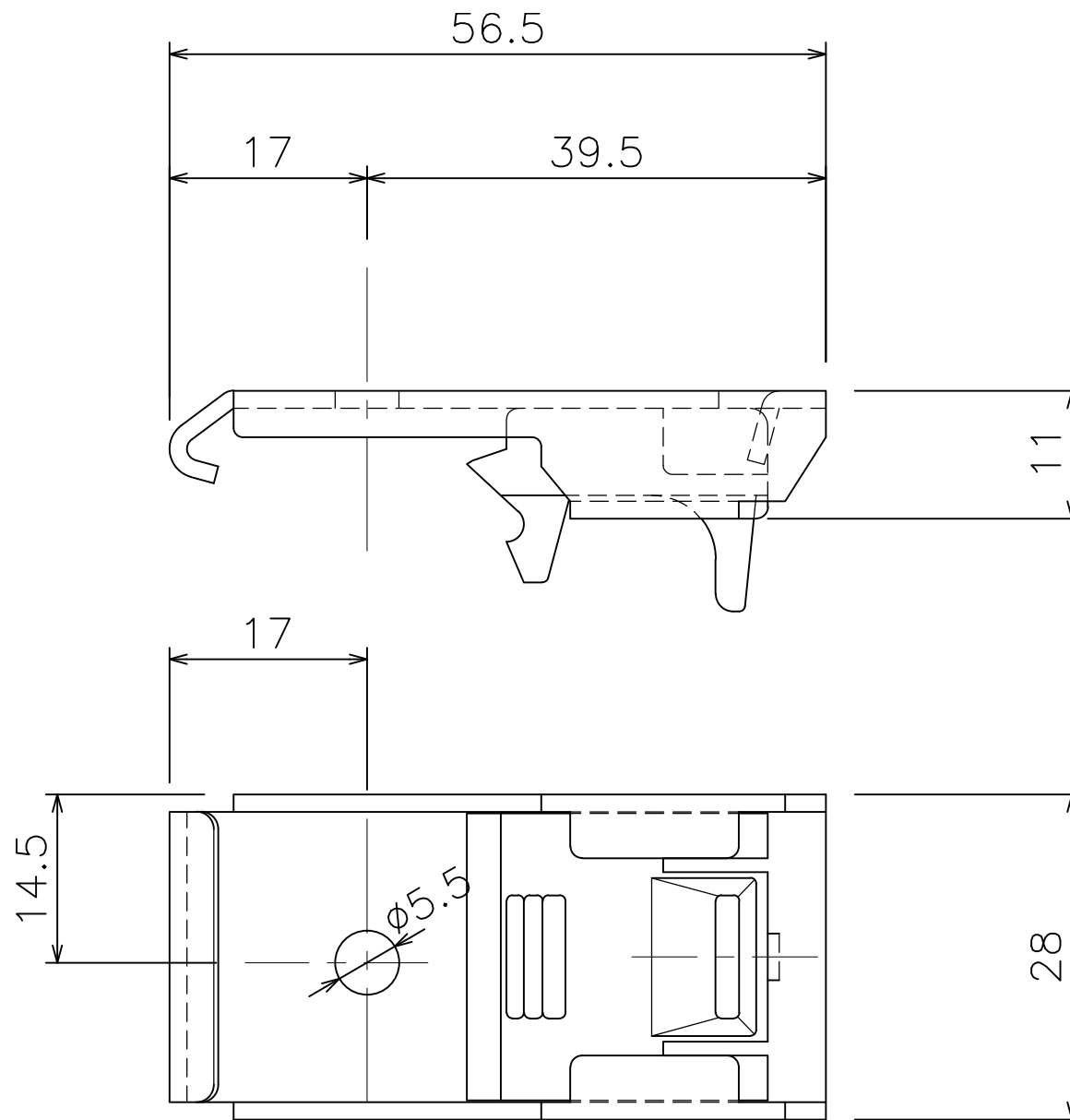
D30 ワンタッチ天井Sブラケット (12T52)
