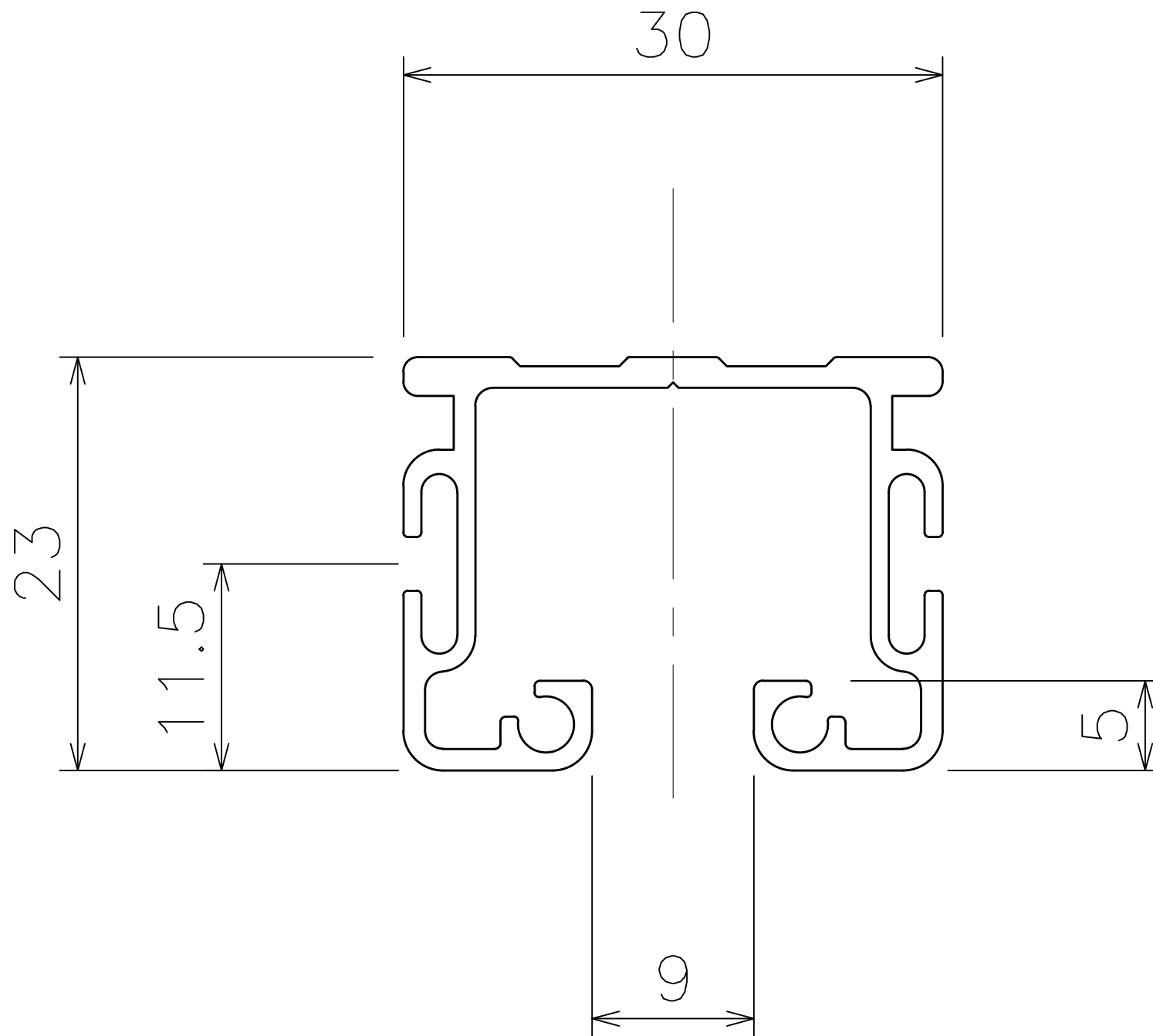
D30隙間シートレール (11L** *-AS)
