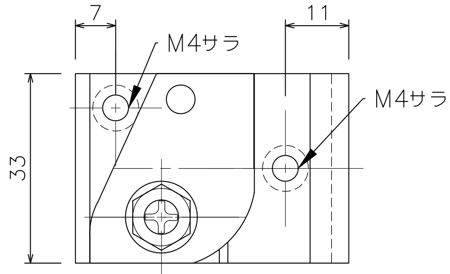
ベンダー 天井先付Sブラケット (19T53)
