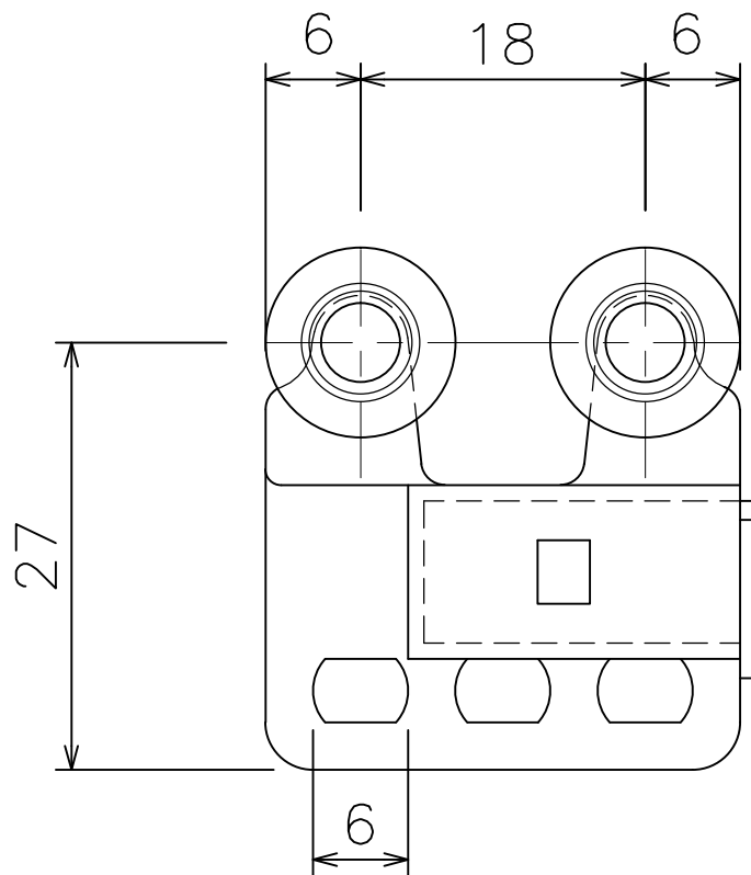
D25 マグネットランナー（片開き）（9T22）
