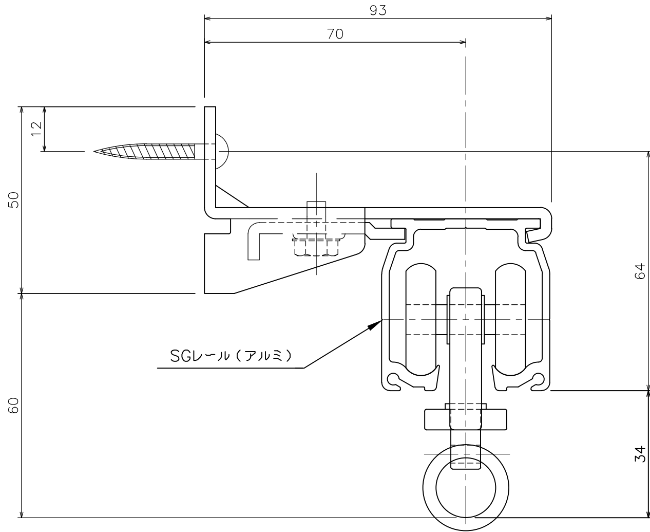
SG Sブラケット (27T41)
