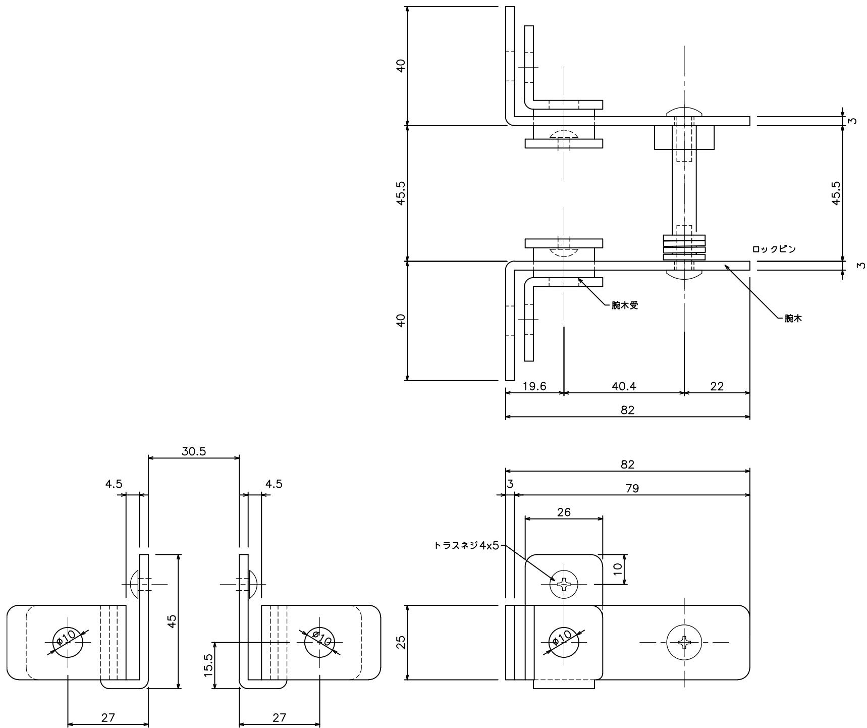
間仕切ロック両開鍵掛穴付 (90T35)
