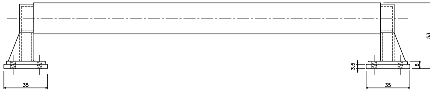
間仕切 ステン大型パイプ取手 (90T68)
