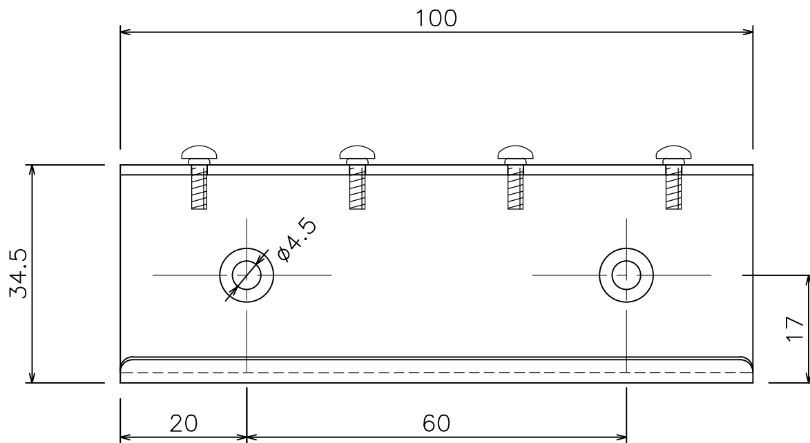
D30 ステンTOPカバー (13T65)
