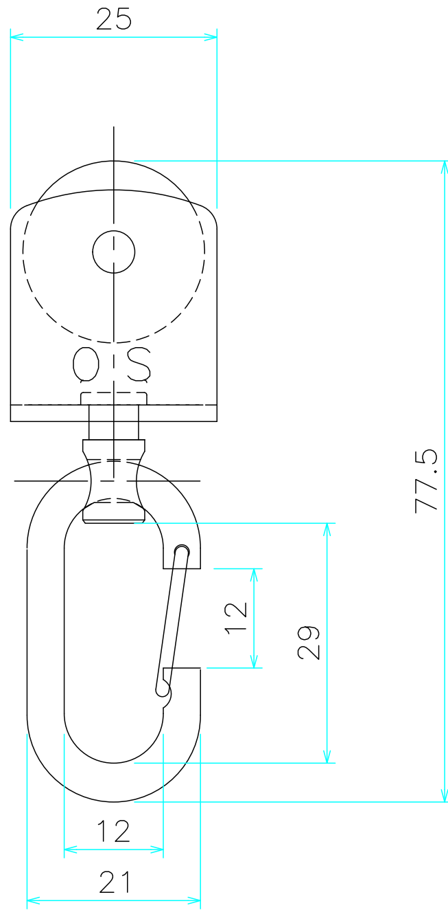
ベンダー ステンワンタッチランナー (19T17)
