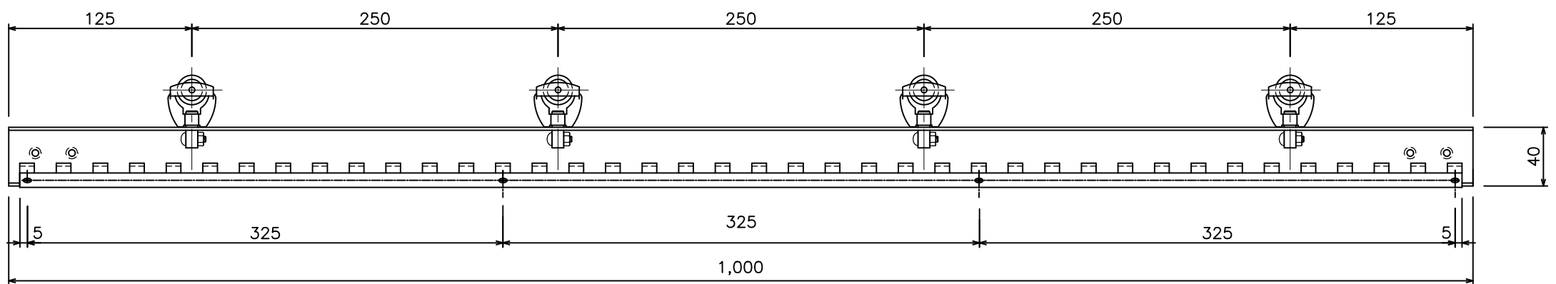
のれんシートフレーム【Aタイプ】可動式スチール寸法図(72A61)
