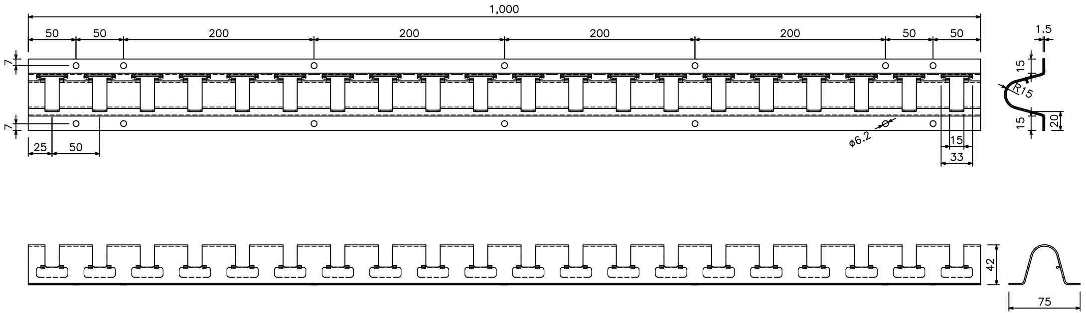
のれんシートフレーム【Bタイプ】ステンレス寸法図(72B12)
