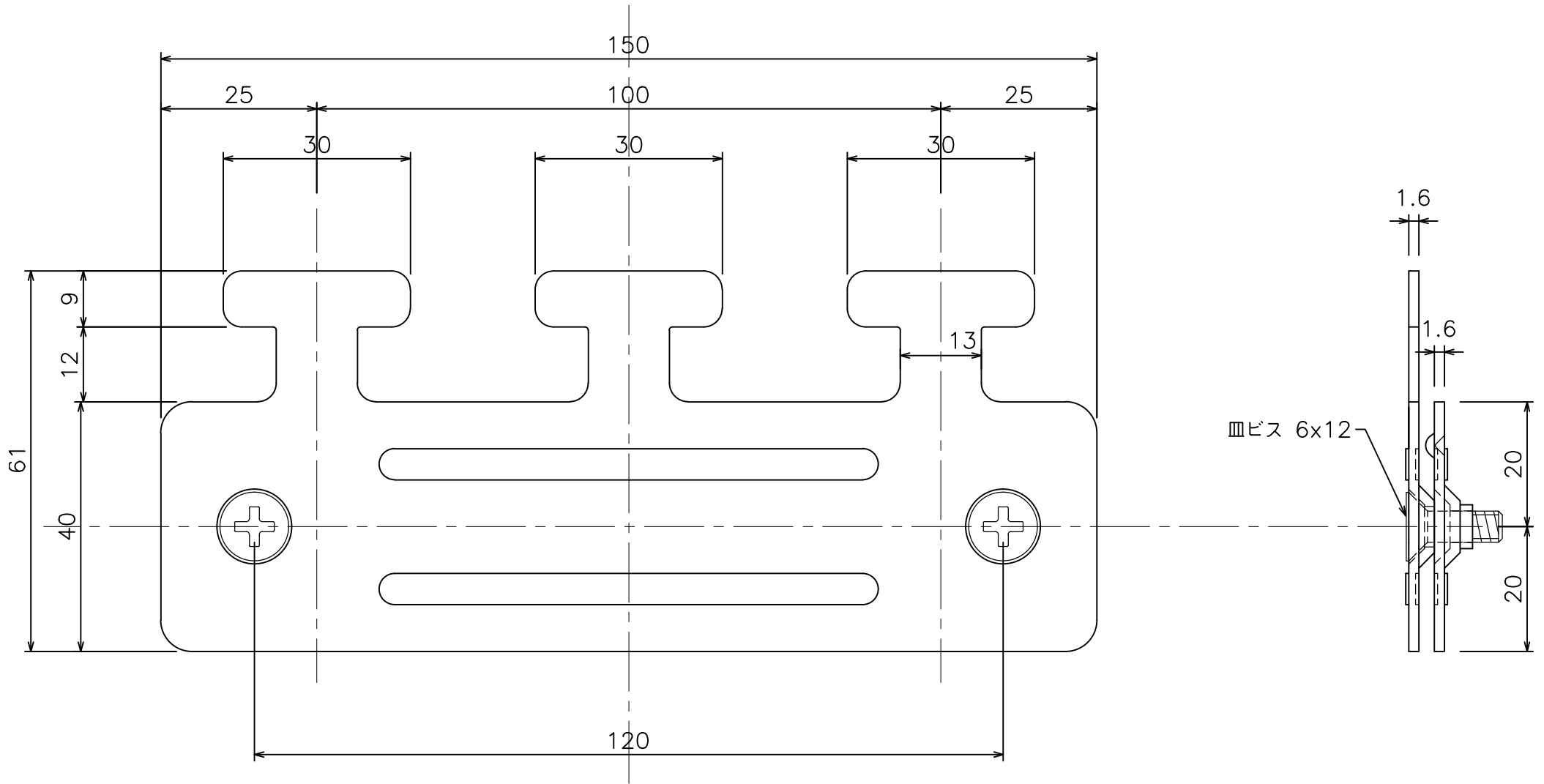
のれんシートハンガー-W200用（スチール）寸法図（72H21）
