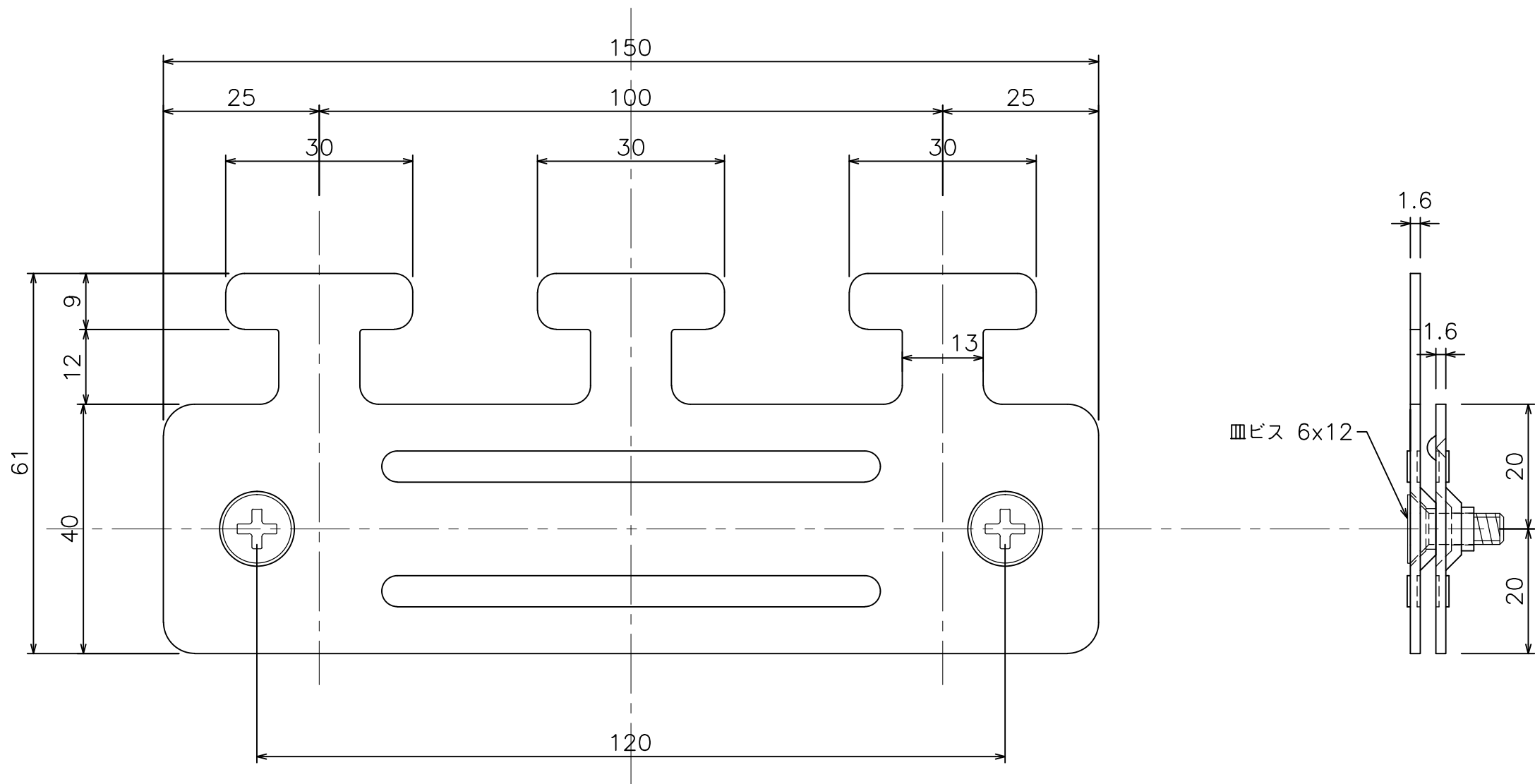
のれんシートハンガ-W200用(ｽﾃﾝ) 寸法図(72H22)
