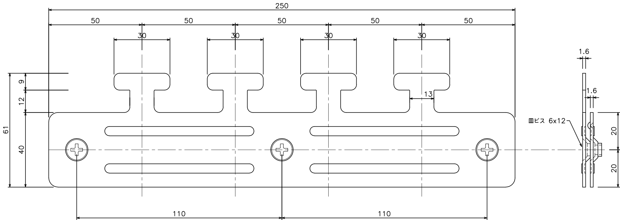
のれんシートハンガ-W300用(スチール)寸法図(72H31)
