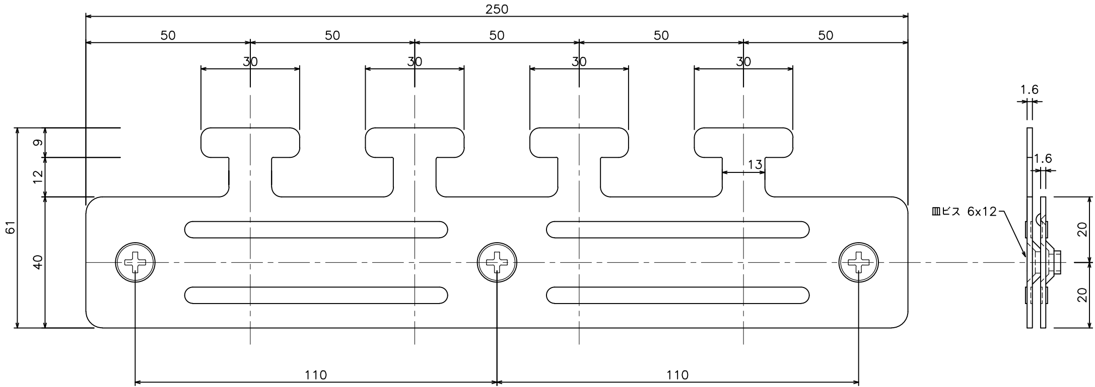
のれんシート用ガ-W300用 (スリ) 寸法図 (72H32)
