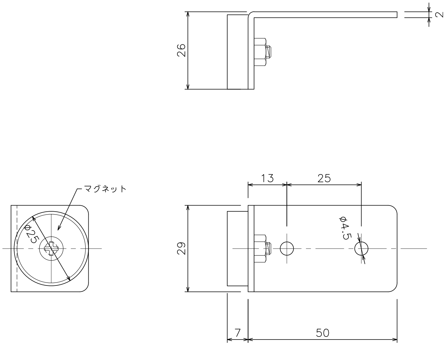
のれんシートフレーム用マグネット寸法図 (72T21)
