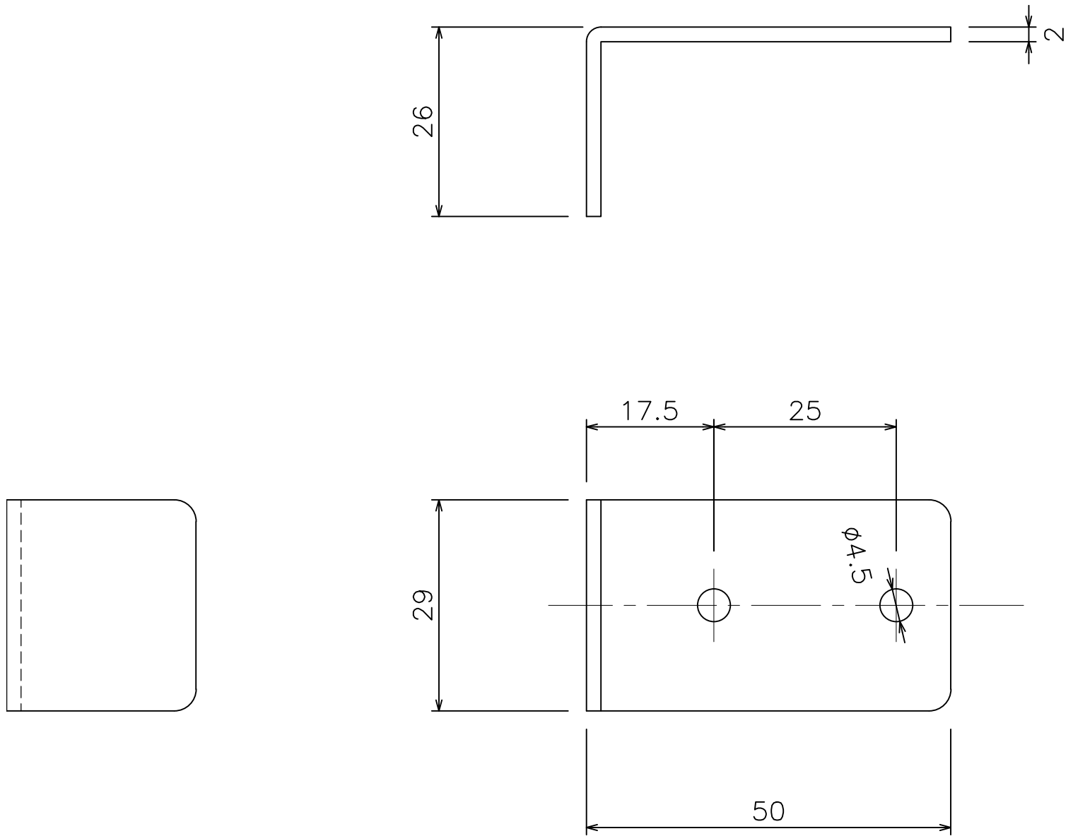
のれんシートフレーム用マグネット受け寸法図 (72T26)
