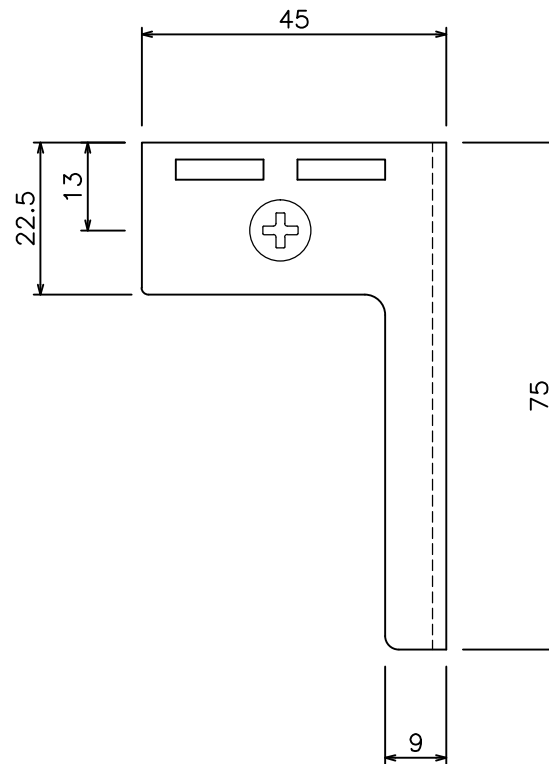
のれんシートフレーム用キャップストップ（スチール）寸法図（72T31）
