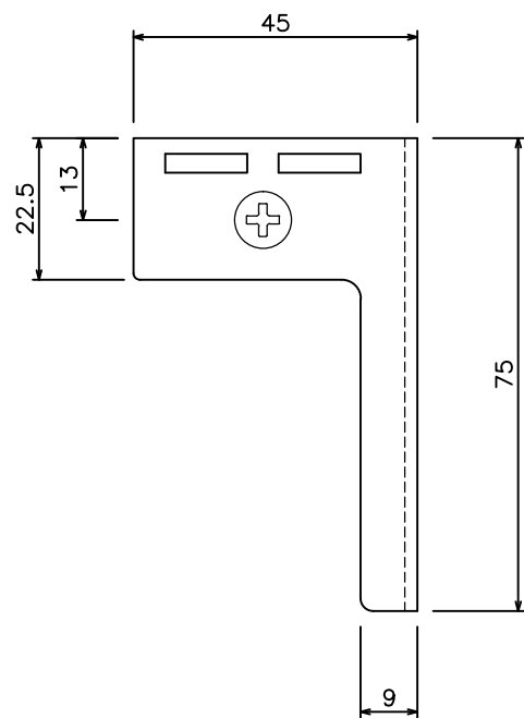
のれんシートフレーム用キャップストップ (ステンレス) 寸法図 (72T32)
