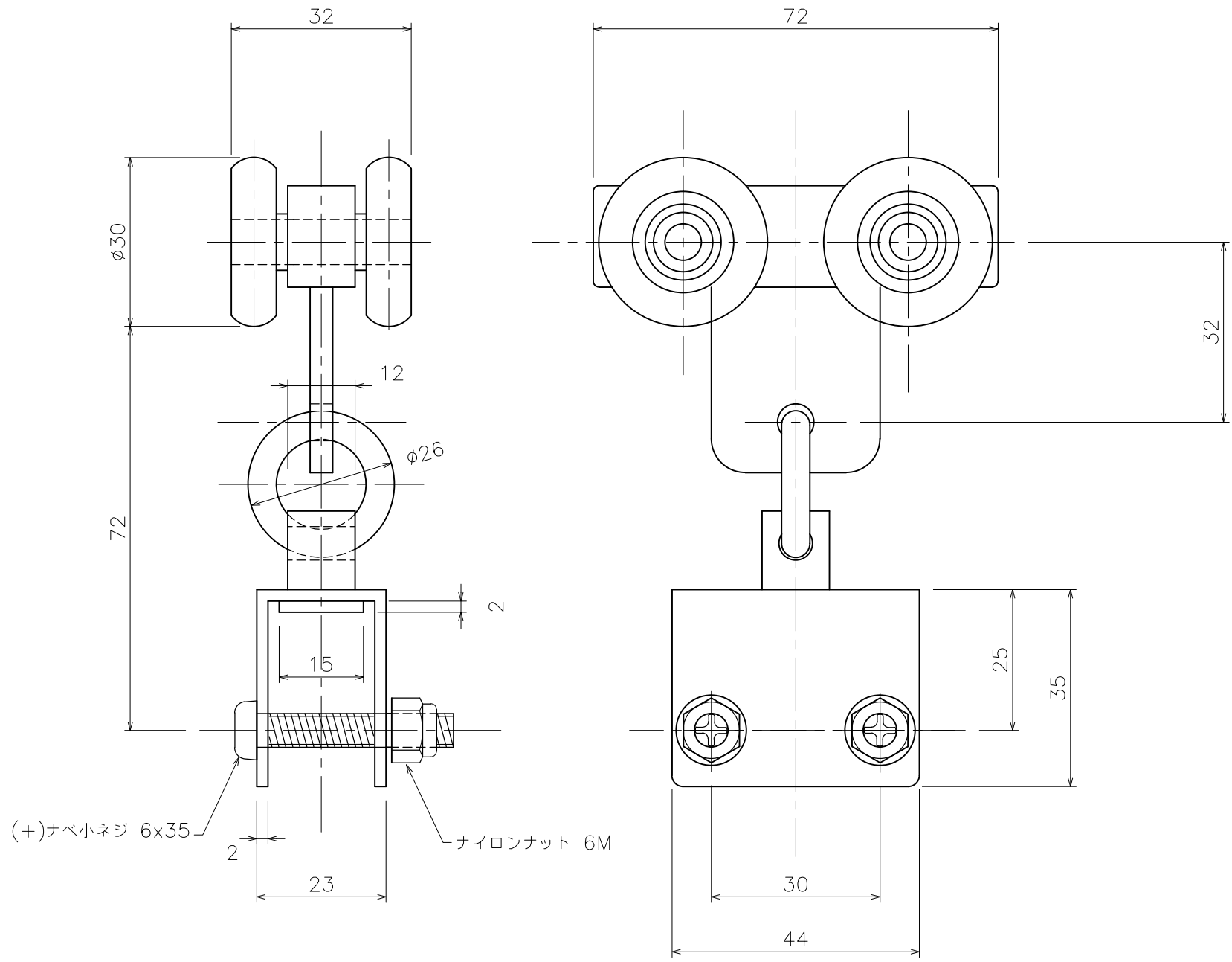
SG 間仕切りランナー (27T28)
