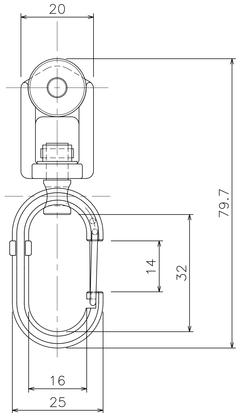
D40 ベアリング入ワンタッチランナー (15T27)
