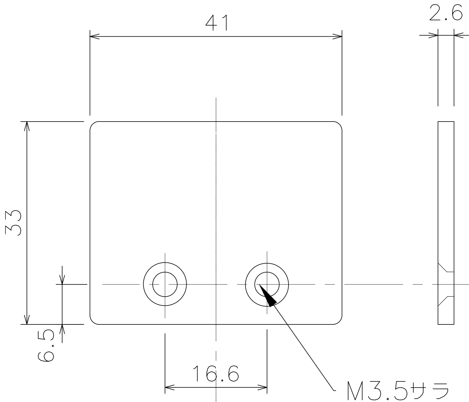
D40 アルミキャッププレート (15T34)
