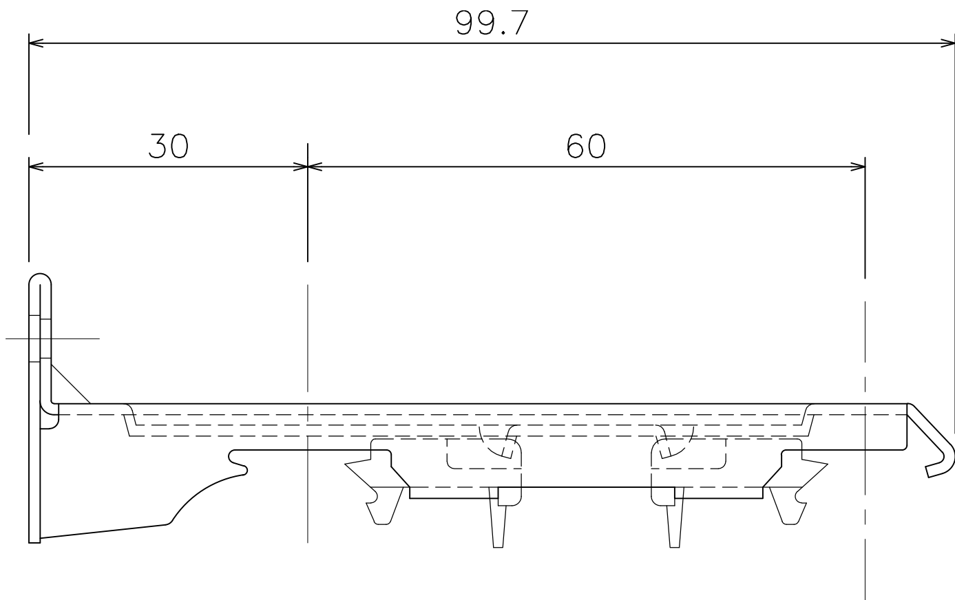
A完全ワンタッチWブラケット (7T42)
