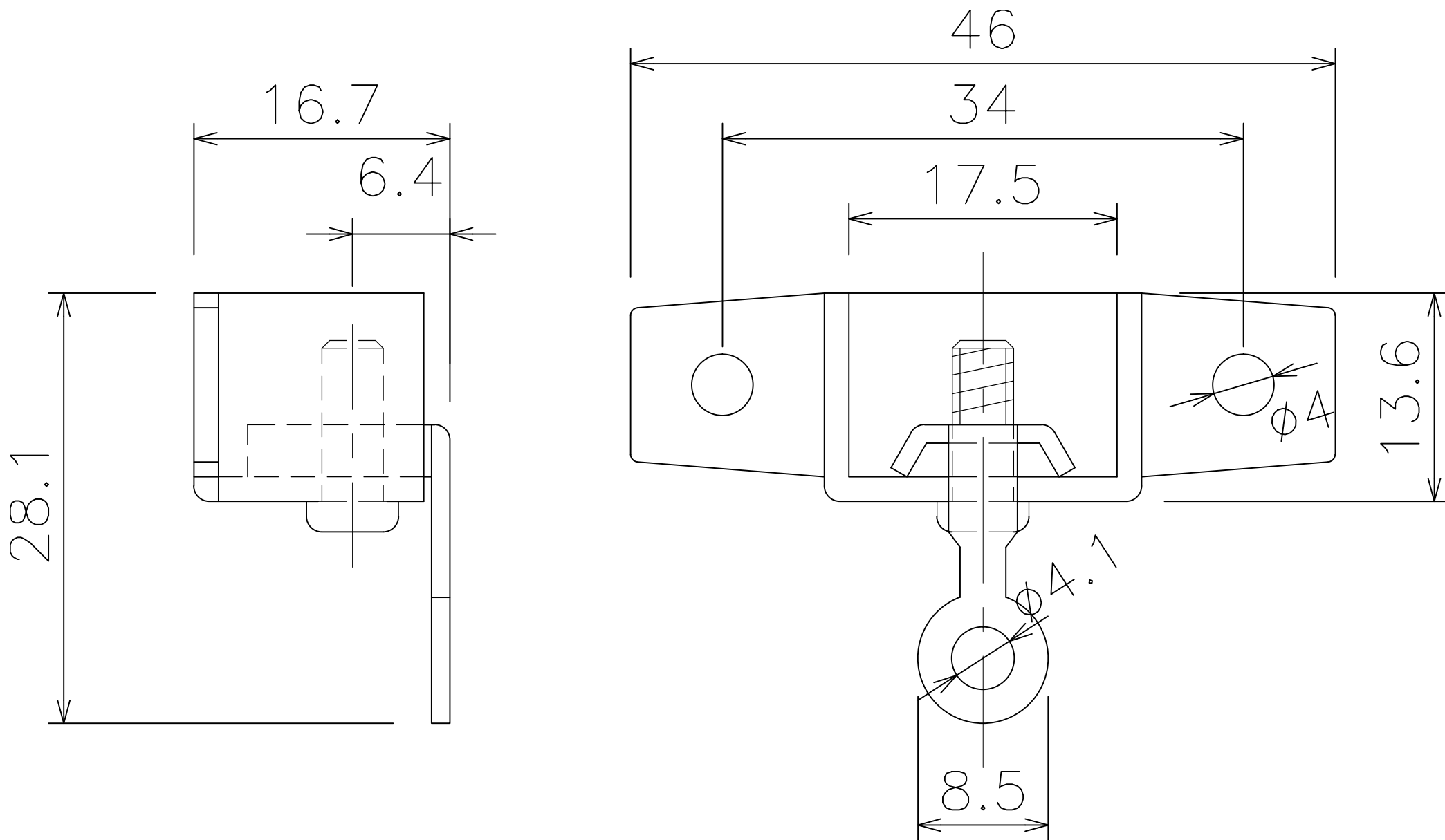
A壁付ソケット (7T36)
