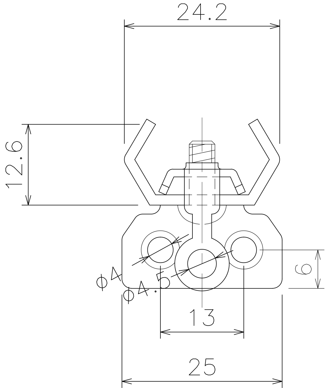
C型 壁付ソケット (ステンレス製) (1T38)
