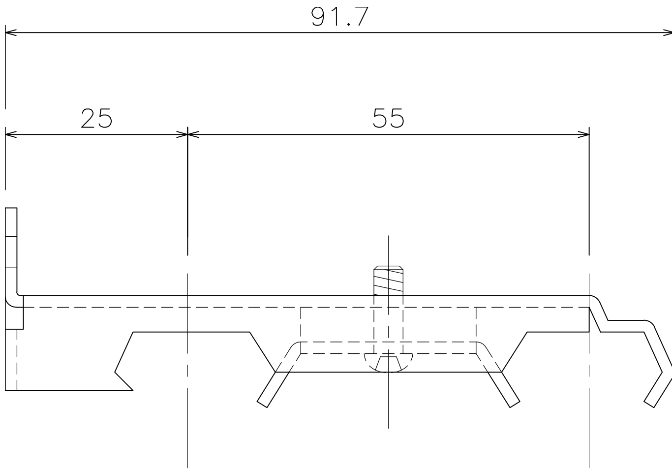
C型 C・Wブラケット (Fタイプ) (1T47)
