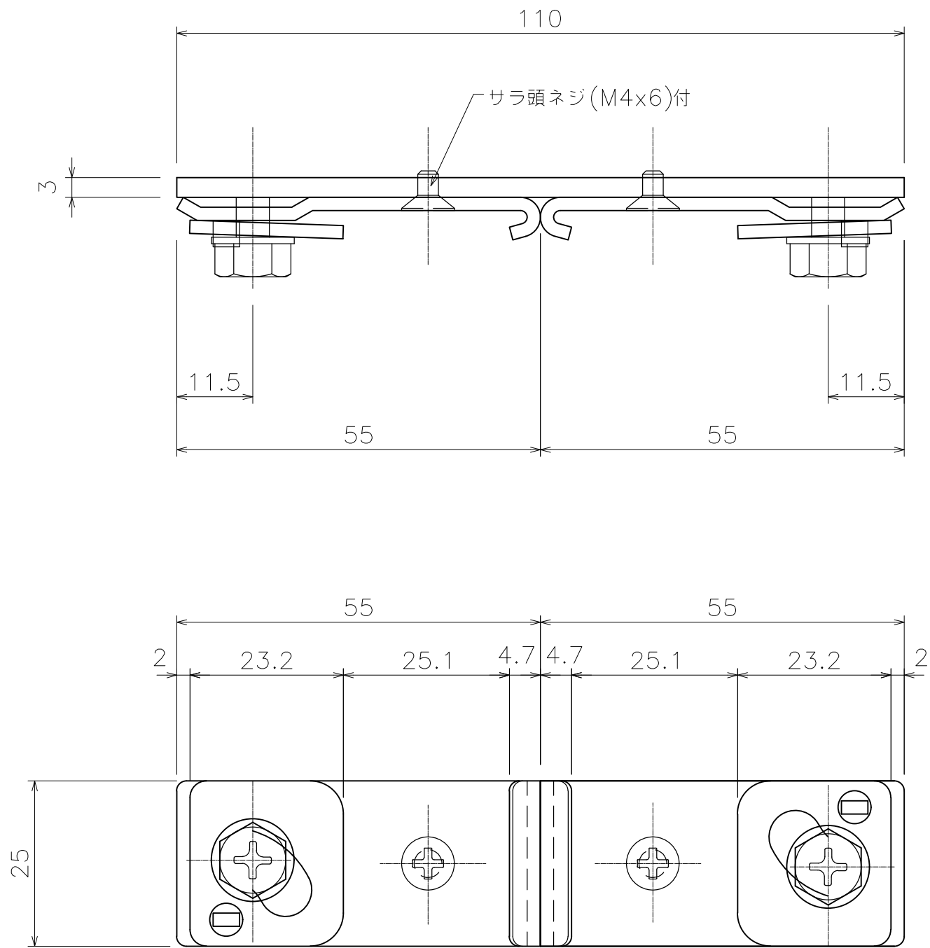
D30天井Wブラケット (12Y13)
