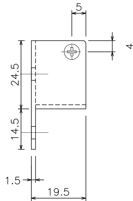
D30 ステン間仕切用壁付ソケット N (13T38)
