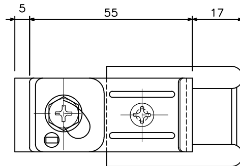
D30 ステンクリップ付天井ブラケット Bタイプ (13Y16)
