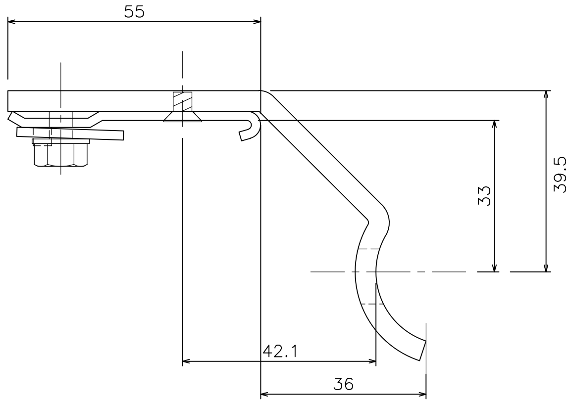
D30 パイプ用ブラケット 32φ (12Y41)
