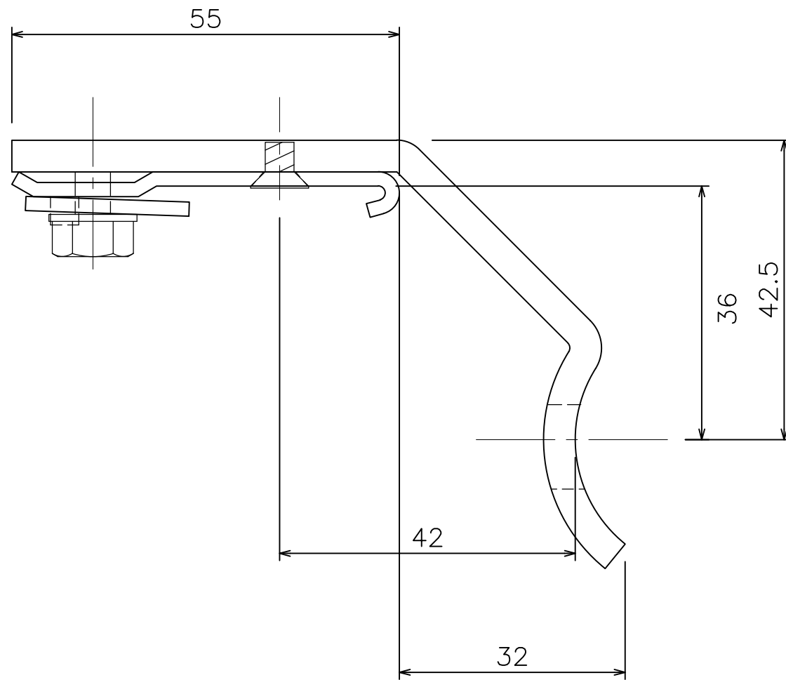
D30 パイプ用ブラケット 38φ (12Y42)
