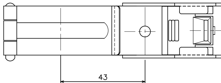
D30 パイプバンド付ブラケット 38Φ用 (12Y47)
