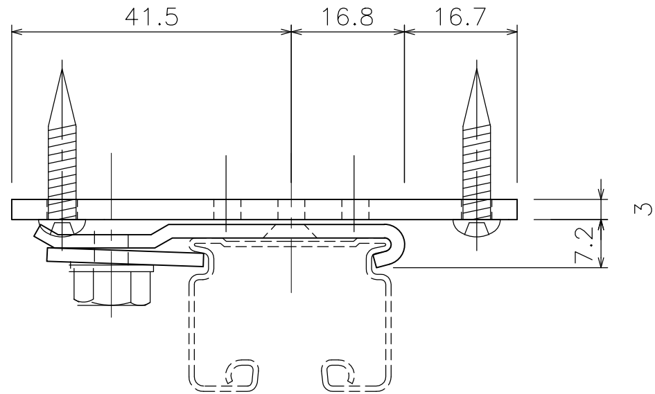
D30天井Sブラケット下地プレート付 (12Y52)
