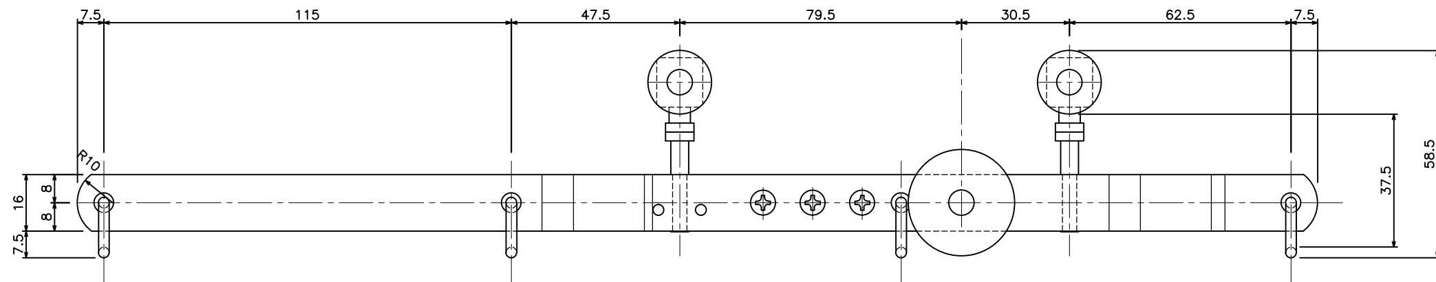
D40 手引用交叉ランナー (15T67)
