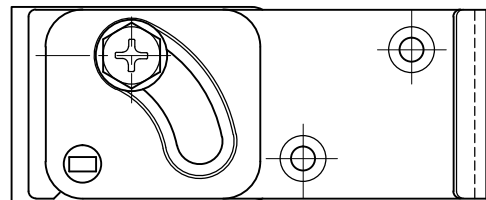
D40 クリップ付天井ブラケット (Aタイプ) (15Y15)
