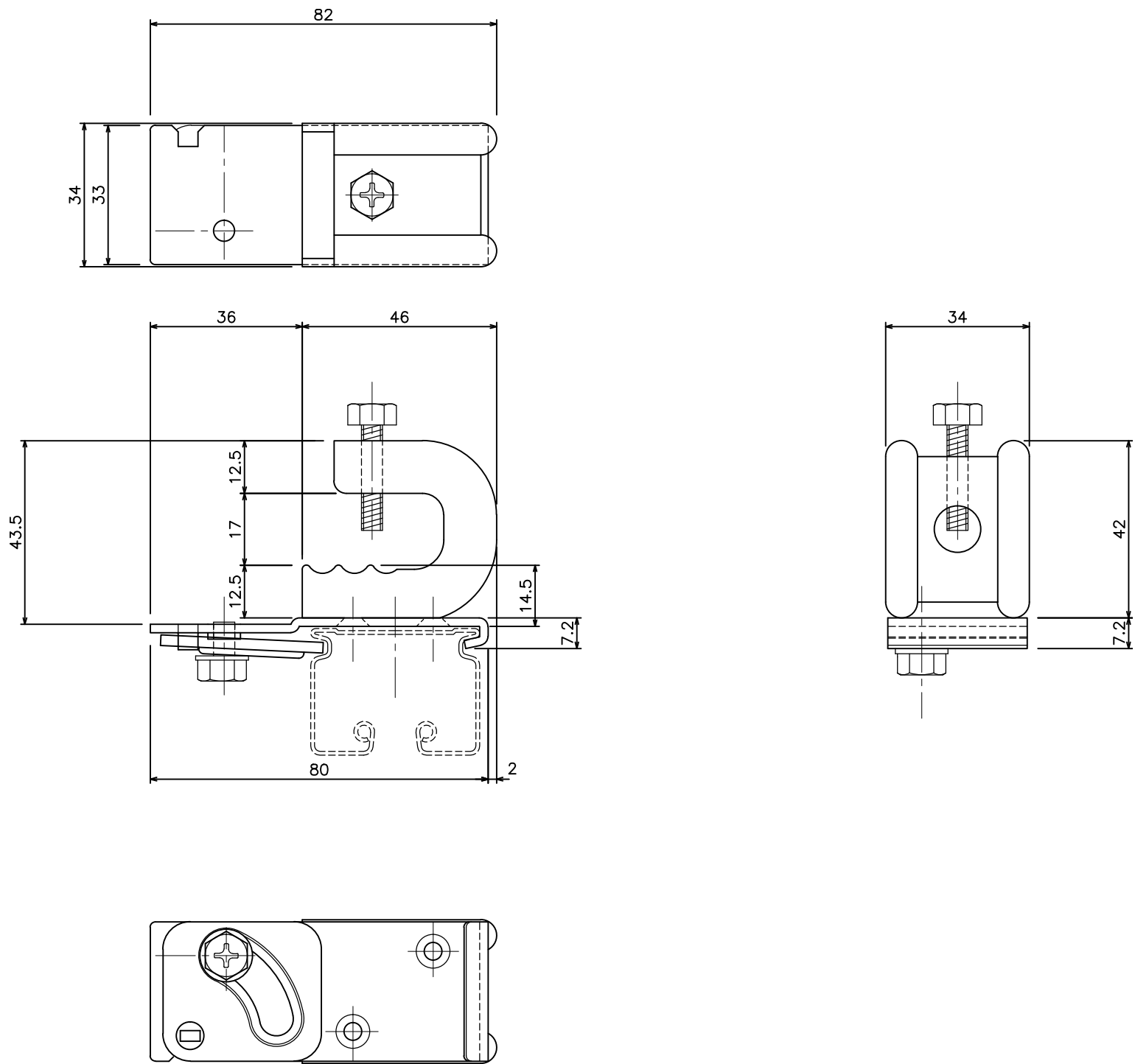
D40 クリップ付天井ブラケット (Bタイプ) (15Y16)
