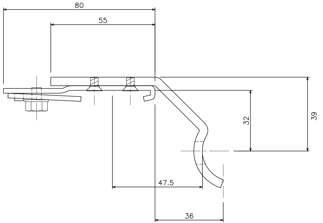
D40 パイプ用ブラケット 32φ (15Y41)
