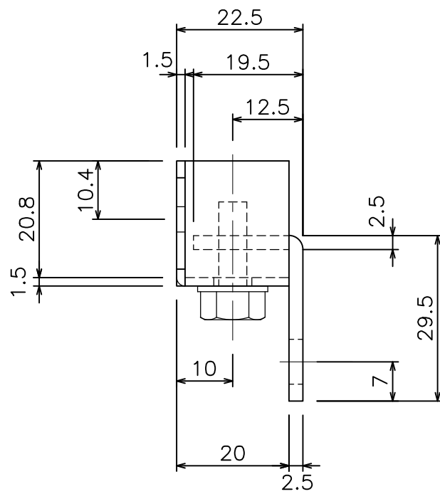
D25 壁付ソケット (9T36)
