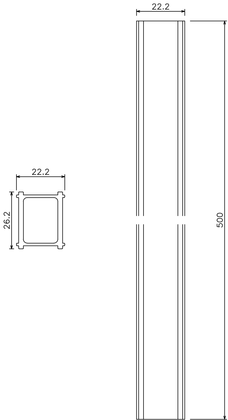
サイドポール【押えバータイプ】 ジョイント (90T96)
