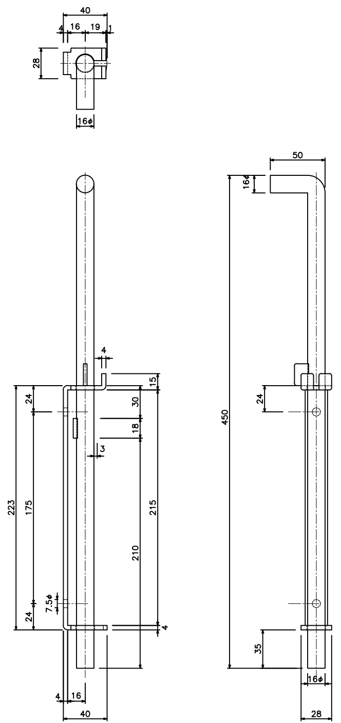
間仕切 ステン落とし16φボルト式 (90T79)
