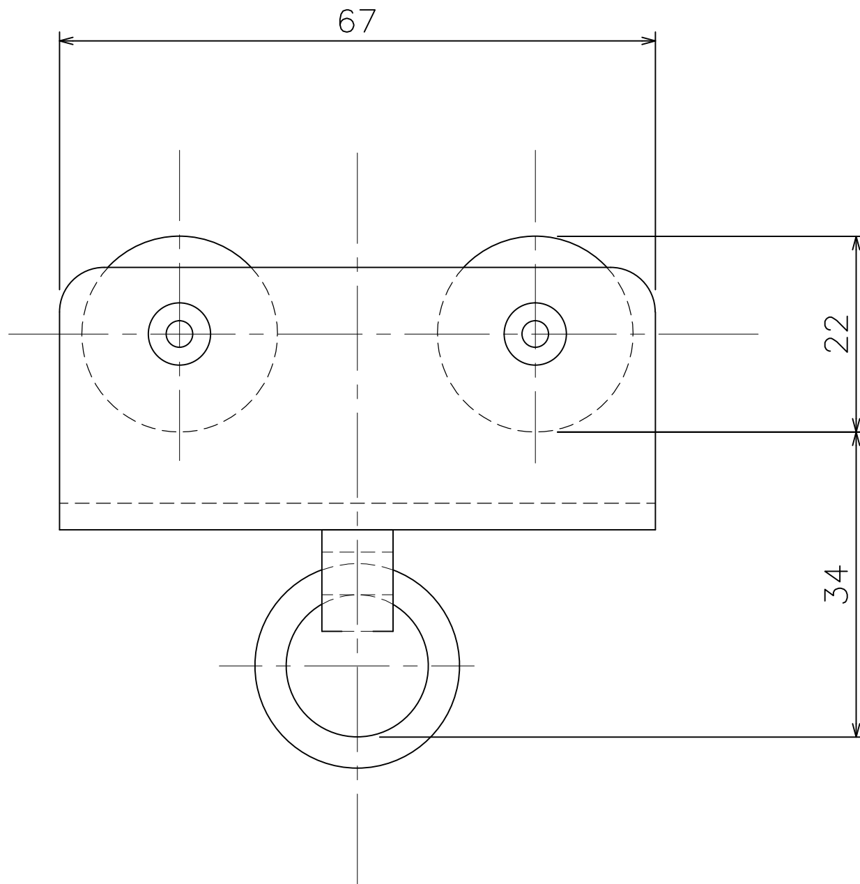
バンダーベアリング入複車ランナー (19T29)
