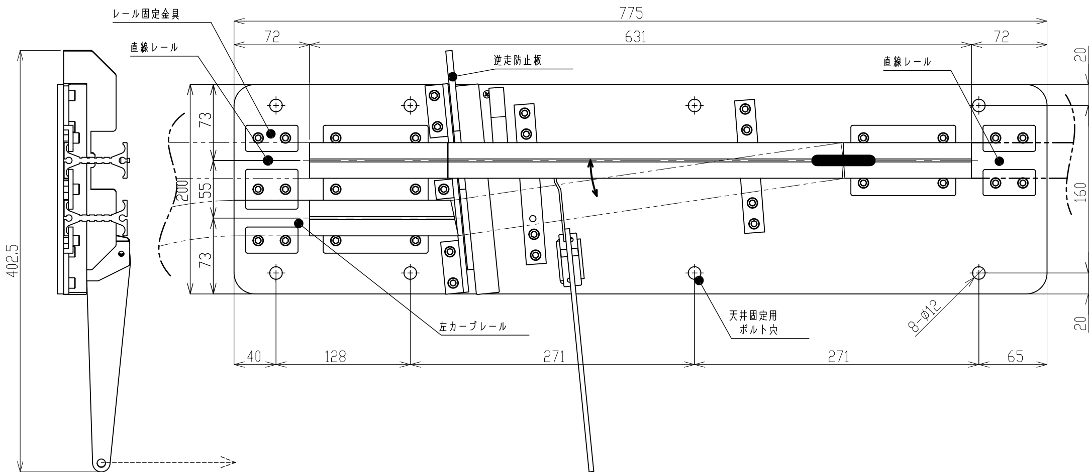
キャリー右分岐ユニット (28L91)
